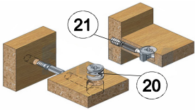
Эксцентриковая стяжка
